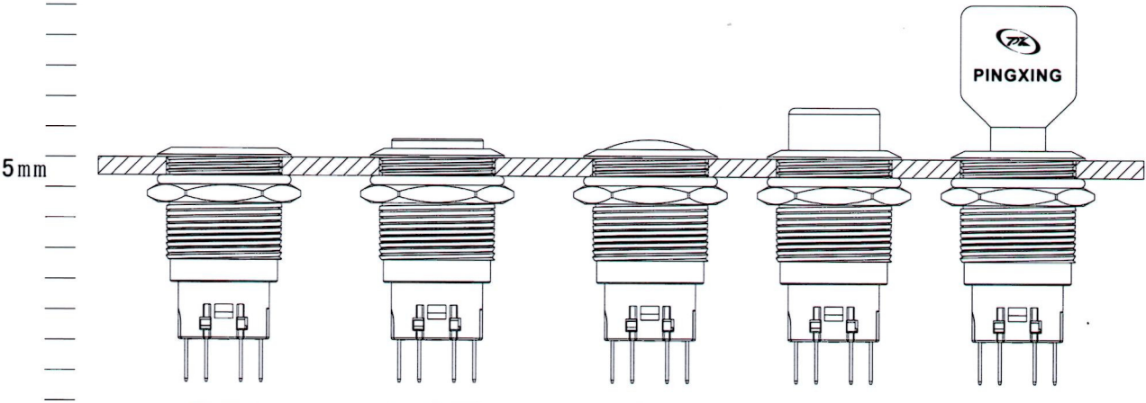
平圆形 P Flat Round Shape 高平圆形 G High flat round shape 球形 Q Ball Shape 旋钮 rotate button 钥匙钮 key button
